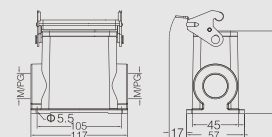
高结构 / High construction
