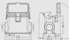
高结构 / High construction
