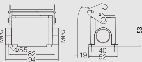
高结构 / High construction
