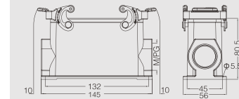
高结构/High construction
