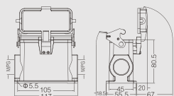
高结构 / High construction
